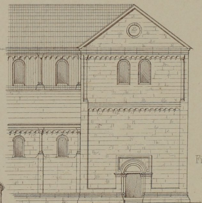
Seitenansicht (System) der Petersbergkirche zu Erfurt (restaurirt-n. Wolfram u.a.)
