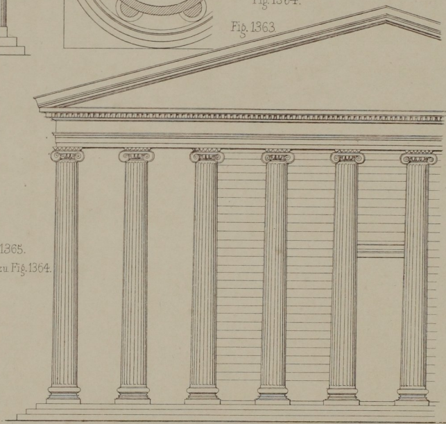
Fig. 1363 Tempel des Apollo Didymaeus bei Milet. (n. Dilletanti) (griech. jon.)
