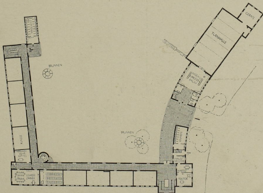
Blick vom Verbindungsgang in den Schulhof. Im Schnittpunkte des Knabenflügels (links) mit dem Mädchenflügel (rechts) der Treppenturm, der eine schnelle Verbindung des Lehrerzimmers mit dem Schulhof herstellen soll. Unten: Erdgeschoß. M. 1:800.
