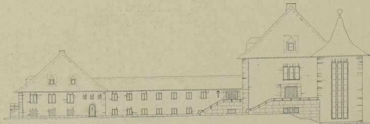
Oben: Südwestansicht des Klassengebäudes mit dem Haupteingang. Unten: Gesamtansicht von Süden. M. 1:600. Links das Turnhallengebäude, in dem am Kopfende die Hausmeisterwohnung untergebracht ist. Die äußeren Wandflächen sind in Ziegelrohbau ausgeführt und geschlämmt; Umrahmung der Eingangstüren, Freitreppe und Sockel in Basallava; Dachdeckung in grauen Handstrichpfannen.
