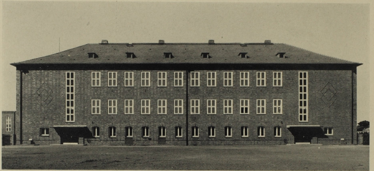
Dreizehnklassige Horst-Wessel-Schule in Guhrau, Regierungsbezirk Breslau. Oben: Ostansicht, vom Schulhof aus gesehen. Unten: Grundrisse und Schnitt. M. 1:600.
