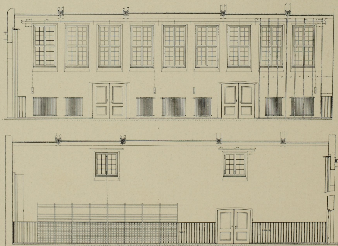
Die Turnhalle der zwölfklassigen Hans-Schemm-Schule in München-Neuharlaching. Zeichnungen im M. 1:120.
