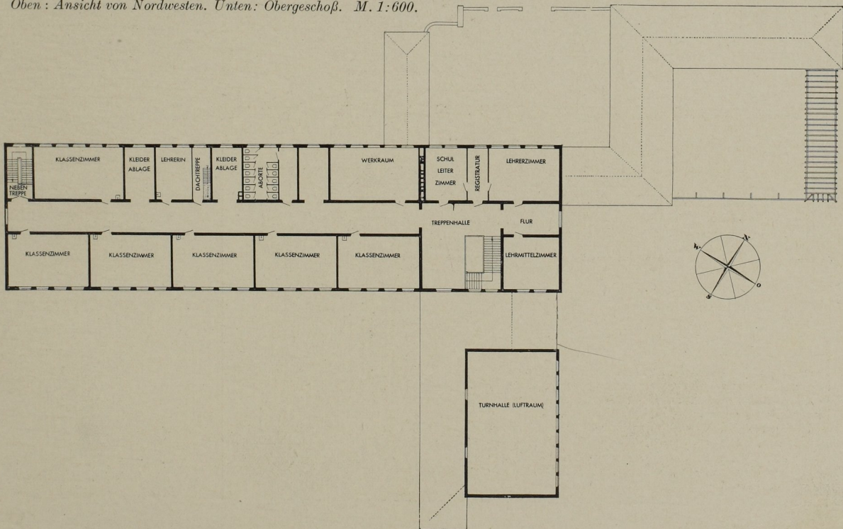
Oben : Ansicht von Nordwesten. Unten : Obergeschoß. M. 1:600.
