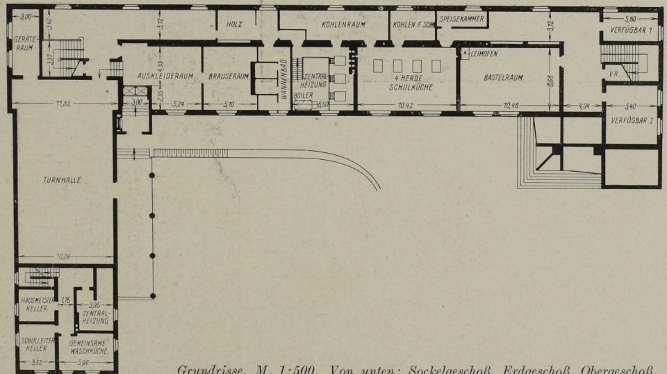
Grundrisse. M. 1:500. Von unten: Sockelgeschoß, Erdgeschoß, Obergeschoß.
