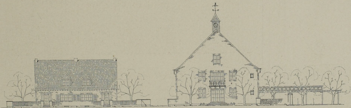
Achtklassige Schule in Köln-Merkenich. Oben: Die Haupttreppe im Erdgeschoß. Hinten die Tür zum Gymnastikraum. Flure und Treppenhaus sind möglichst licht gehalten. Unten: Die Hauptschaufseiten des Klassenhauses und des Rektor- und Lehrerwohnhauses. M. 1:400.
