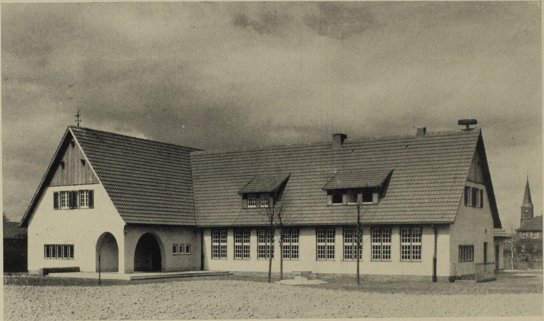
Vierklassige Schule in Mecklenbeck, Regierungsbezirk Münster. Architekt: Stadtbaumeister Friedrich Schmeißer, Münster. Oben: Ansicht von Südosten. Unten: Grundriß. M. 1:300.
