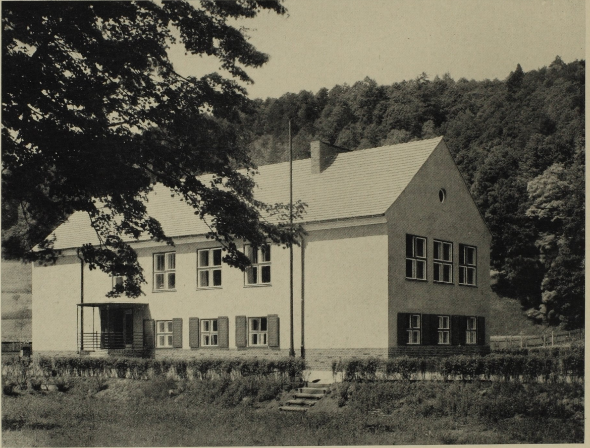
Dreiklassige Schule in Ober-Weistritz, Regierungsbezirk Breslau. Architekt: Ernst Pietrusky, Breslau. Oben: Die Haupteingangsseite. Die Außenflächen sind über dem Klinkersockel hell verputzt; das Dach ist mit grauen Biberschwänzen eingedeckt. Unten: Erdgeschoß. M. 1:300.
