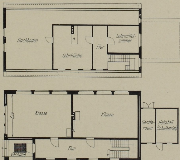
Erdgeschoß und Dachgeschoß des Schulgebäudes. M. 1:300.
