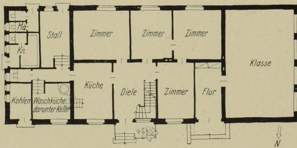
Einklassige Schule bei Stadthorn, Regierungsbezirk Münster. Architekt: Preußische Staatshochbauverwaltung. Grundriß und Südansicht. M. 1:300.
