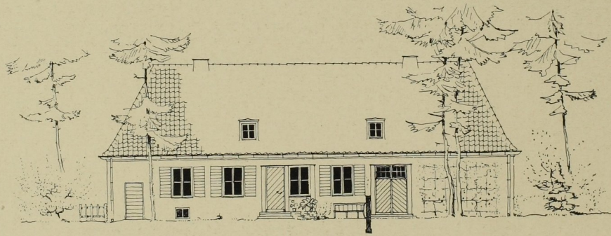
Einklassige Schule bei Stadthorn, Regierungsbezirk Münster. Architekt: Preußische Staatshochbauverwaltung. Grundriß und Südansicht. M. 1:300.
