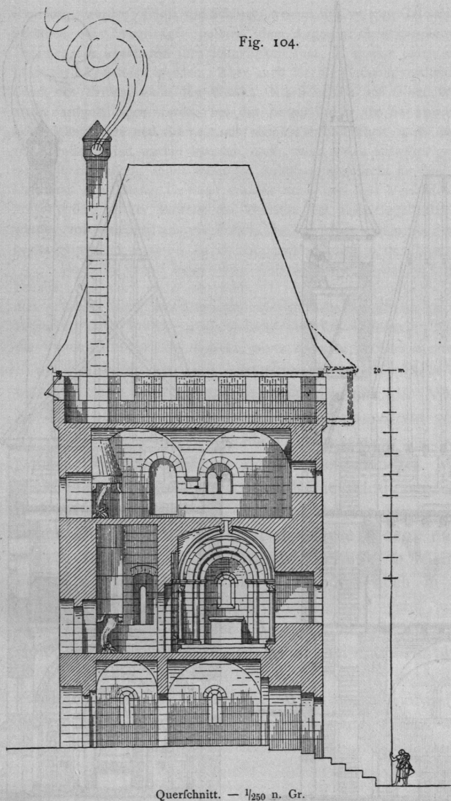
Querchnitt. — 1/250 n. Gr.
