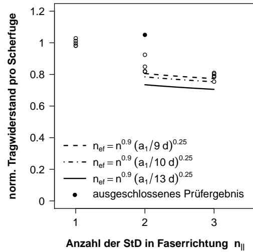
Abb. 6.4.9: Normierter Tragwiderstand pro Scherfuge F_{v,nrm} versus Anzahl der Stabdübel in Faserrichtung n_{\parallel}
