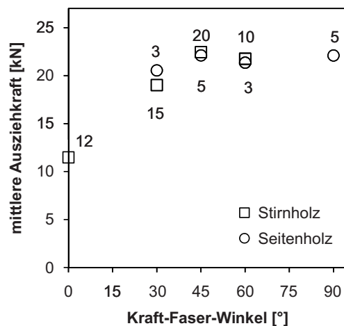
Abb. 4.2.1: Ausziehfestigkeit von SFS WT-T 8,2 × 300 bei einer effektiven Einschraublänge von l_{\text{ef}} = 130 mm – 6 mm in Fichtenholz mit \rho_{12} = 455 kg/m 3 bei u = 14,4\%
