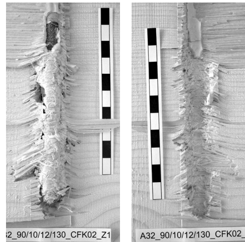
(b) Probekörpern der Serie „zurückgesetzter Verbund“ mit zähmodifiziertem Klebstoff nach Pörtner und Seim (2008)
