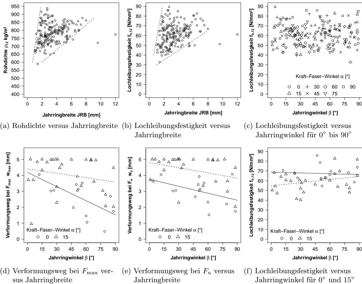
Abb. 5.5.1: Streudiagramme zum Einfluss der Jahrringe auf die Lochleibungsfestigkeit und die Verformungswege des Eschenholzes bei Stabdübeln mit 12 mm Durchmesser
