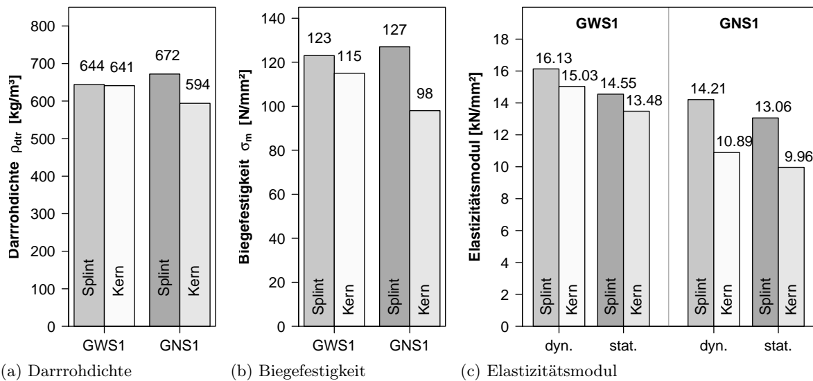
Abb. 1.4.3: Mittlere Darrohndichten, Biegefestigkeiten und Elastizitätsmoduln in Splint- und Kernholz der Untersuchungskollektive GWS1 und GNS1 nach Oliver-Villanueva (1993, S. 107 und 135)
