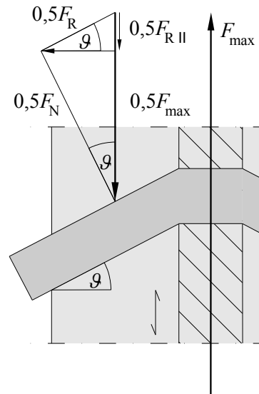
Abb. 6.4.7: Reibungskraft bei Stabdübelverbindungen
