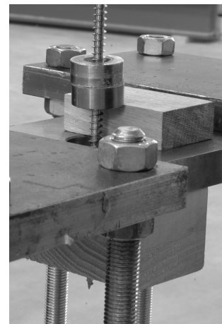
(c) Probekörper mit durchgeschraubter Holzbauschraube
