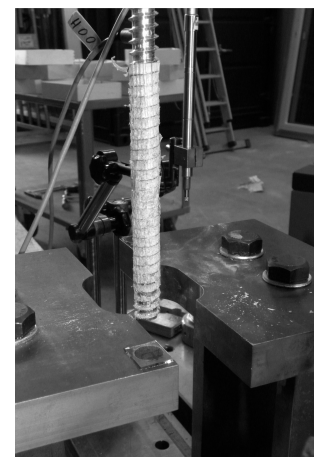
(c) Nach Prüfung mit Einschraubwinkel 90^\circ
