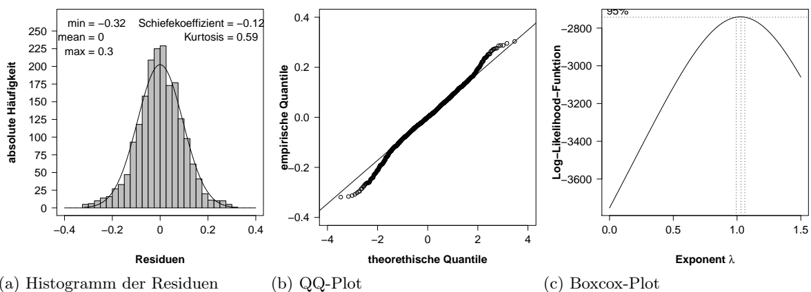
Abb. 4.8.14: Histogramm der Residuen, QQ- und Boxcox-Plot für Modell nach Gleichung (4.117)
