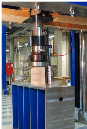
(a) Prüfgerüst mit seitlich gehaltenem Prüfzylinder und quaderförmigen Probekörper
