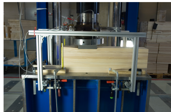
(e) Deformierte Schwelle mit beidseitigem Vorholz unter Lasteinleitungsplatte und Kugelkalotte
