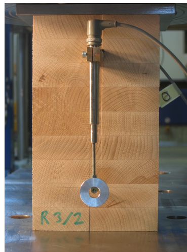
(b) Quaderförmiger Probekörper aus Buchen-Rift BU_R3_2
