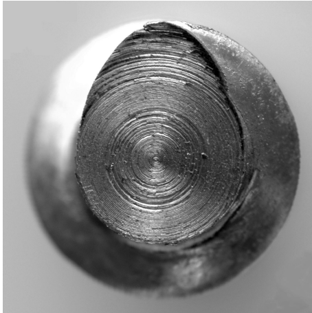
(a) Foto des abgedrehten Querschnitts
