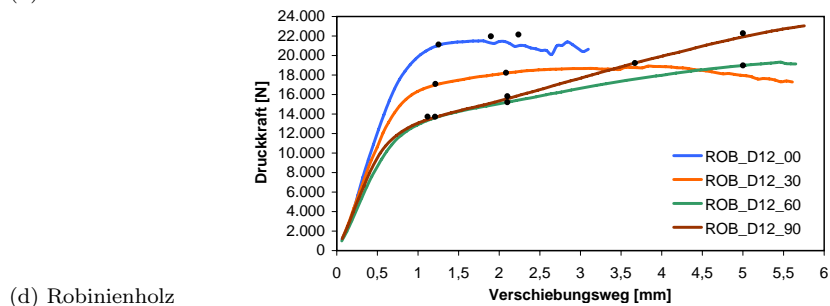
Abb. D.4.3: Gemittelte Last-Verformungs-Kurven der Lochleibungsversuche bei verschiedenen Holzarten und Durchmesser 12 mm
