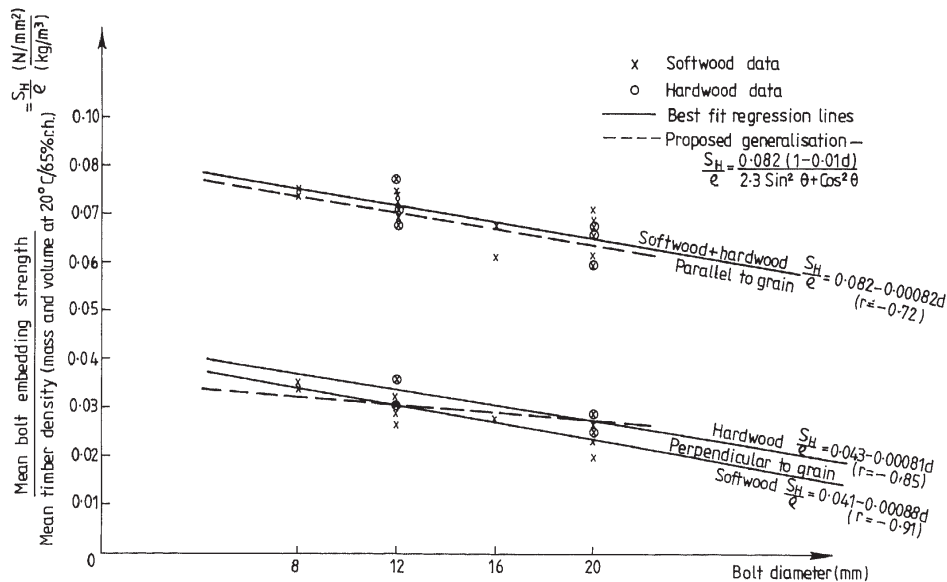
Abb. 5.1.3: Auf die Normalrohldichte bezogene Lochleibungsfestigkeit versus Durchmesser aus Whale und Smith (1986b)
