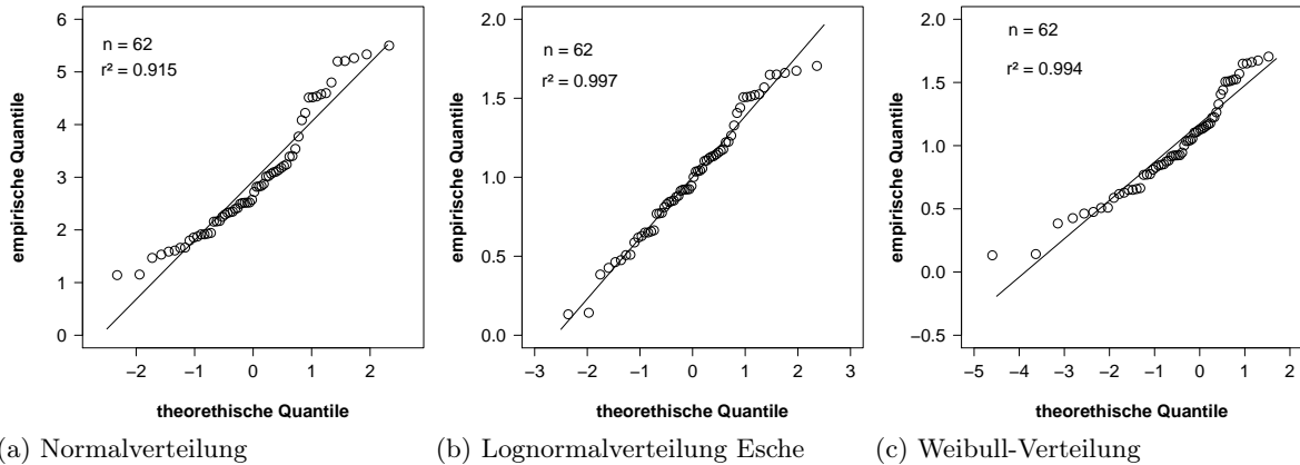
Abb. 3.4.4: QQ-Diagramme der Querzugfestigkeit von Eschen-BSH bei Normal-, Lognormal- bzw. Weibull-Verteilung
