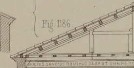
Geschlossener Dachstuhl v. S. Paolo Fuori Le Mura. (n. Hübisch.)
