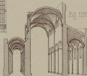
Romanisches Gewölbesystem. (n. W. Lübke.)
