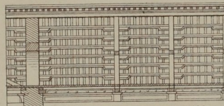
Fig. 1187. Längenschnitt zu Fig. 1186.
