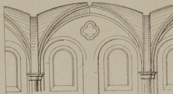
Fig. 1196. Romanisches Gewölbe (Dom zu Worms).
