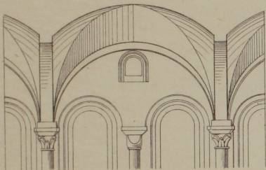
Fig. 1198. Romanisches Gewölbe. (Dom zu Speier).
