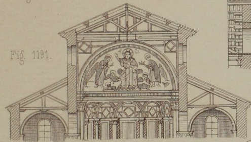
Offener roman. Dachstuhl v. S. Miniato zu Florenz.
