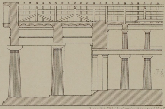
Siehe Fig. 1161. (Längenschnitt) (circa 430 v. Chr.)
