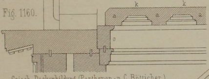
Griech. Deckenbildung (Parthenon - n.C. Bötticher)
