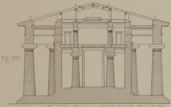
Tempel zu Pastum (griech-dorisch) (Querschnitt).
