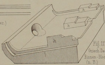
Fig. 1165. (Gr.) Unteres Dachende.
