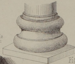
Romanische Säulenbasis (Kz. Ottmarsheim XI. Jahrh. (n. W. Lübke.)
