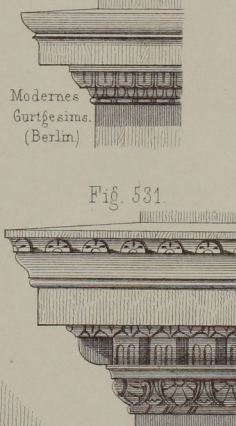
Modernes Gurtgesims.
