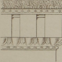
Fig. 406. Römisch-Korinth. Gebälk v Tempel d. Jupiter Römisch-Korinth. Hauptgesims v Tempel d. Jupiter Stator zu Rom (S. Stegmann)
