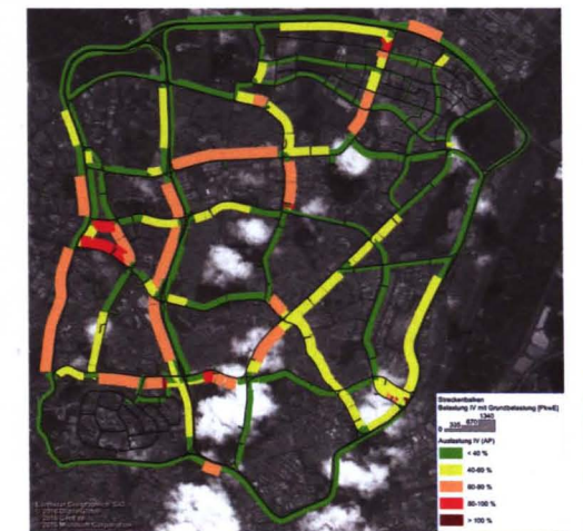
Abbildung 5: Simulation einer Steuerungs- variante für ein Teilnetz von Singapur.
