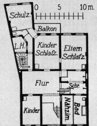
WOHNHAUS BEHRENSTRASSE 6. GRUNDRISSSE DES ERSTEN UND ZWEITEN OBERGESCHOSSES.
