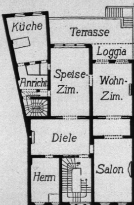
WOHNHAUS BEHRENSTRASSE 6. GRUNDRISSSE DES ERSTEN UND ZWEITEN OBERGESCHOSSES.
