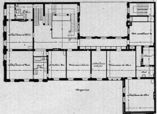
WOHNHAUS MATTHÄIKIRCHSTRASSE 31 BIBLIOTHEK. GRUNDRISSSE DES ERD- UND OBERGESCHOSSES.
