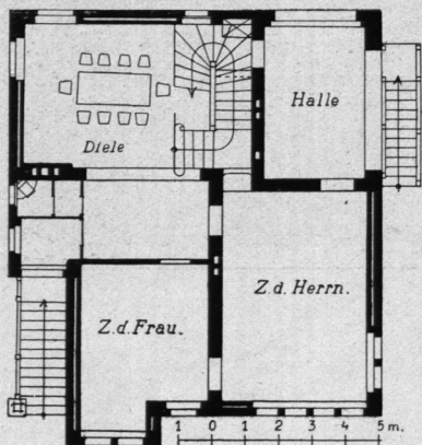
VILLA BRAUN IN VILLENKOLONIE GRUNEWALD. GRUNDRISSE DES ERD- UND OBERGESCHOSSES.
