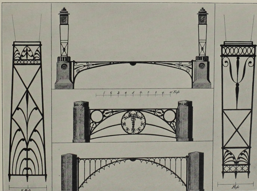
Eisengegossene Rampen an der ehemaligen Kgl. Bibliothek und ehemals am Lustgarten Laternenständer. Schlesischer Eisenguß um 1800
