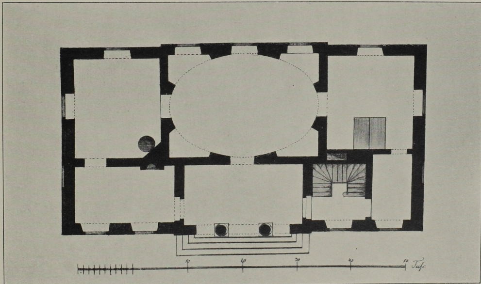
Gartengebäude. Entwurf von C. F. Langhans d. J. Berlin 1797
