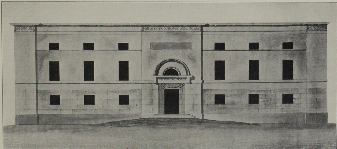
Aufrisse der Vorder- und Seitenfassade des Königsberger Theaters. 1799. Nach Fr. Gillys Plänen kopiert
