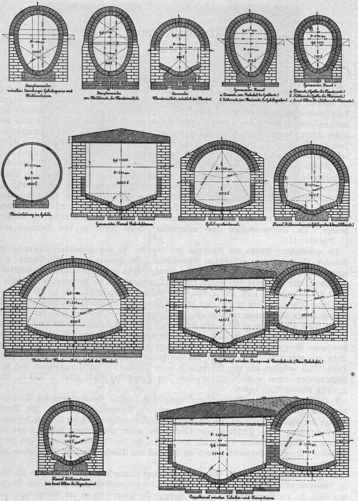
Abb. 1292 bis 1304. Kanalquerschnitte.
