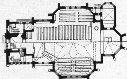
Grundriß.
