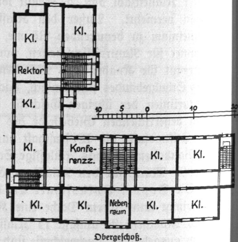
Abb. 1081. Volksschule Herderstraße.
