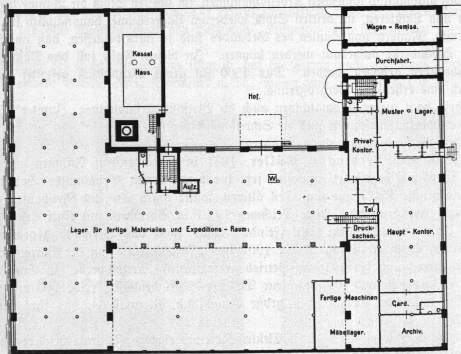
Abb. 901 und 902. Nähmaschinenfabrik Guhl & Harbeck, Querschnitt und Grundriß.
