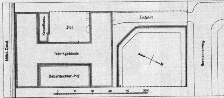
Abb. 900. Nähmaschinenfabrik Guhl & Harbeck, Lageplan.
