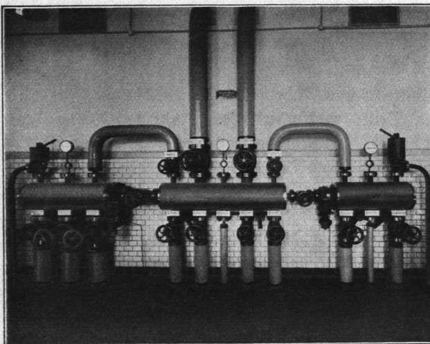
Abb. 896. Rud. Otto Meyer, Dampfverteilungsstelle in einer Heilanstalt.
