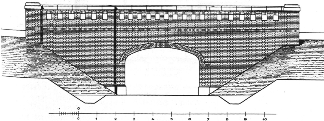
Abb. 845. Walddörferbahn, Wegunterführung in dem Haselhorst (Volksdorf).
