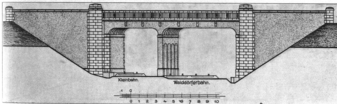
Abb. 844. Walddörferbahn, Überführung des verlegten Bergstedter Weges (Volksdorf).
