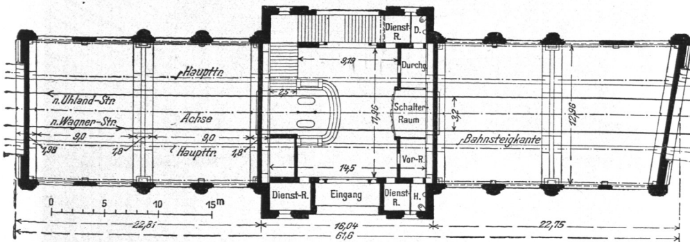
Abb. 825. Haltestelle Mundsburg, Grundriß des Bahnhofsgebäudes.
