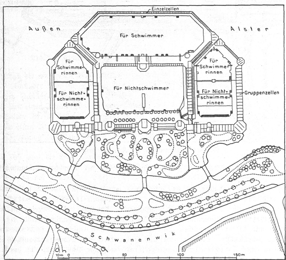
Abb. 762. Badeanstalt Schwanenwik, Lageplan.
