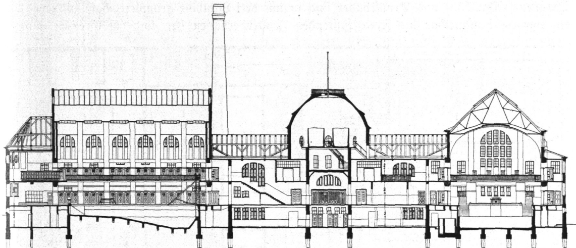
Abb. 751. Badeanstalt Hammerbrook, Längenschnitt.
