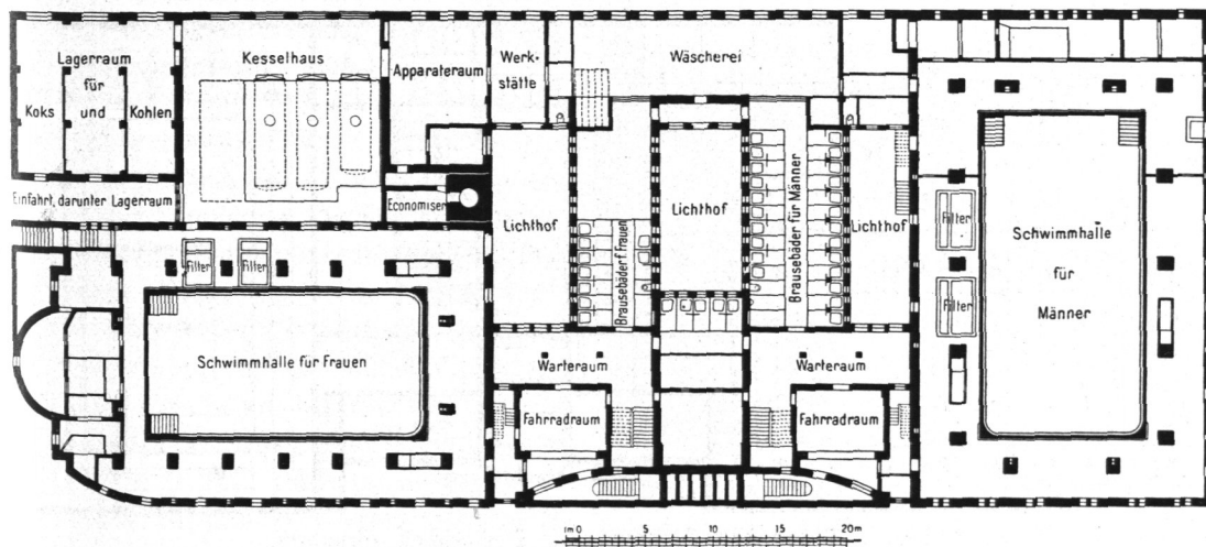
Abb. 752. Badeanstalt Hammerbrook, Kellergeschoß, Grundriß.
