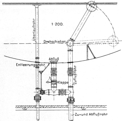
Abb. 736. Zu- und Abflusseinrichtungen der Hochbehälter.
