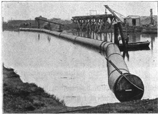
Abb. 726. Verlegung des den Elbe-Bille-Kanal durchziehenden Dükers.
