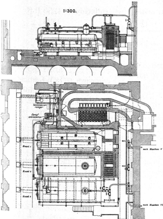
Abb. 707. Dampfkeffelanlage der Maschinen V und VI.
