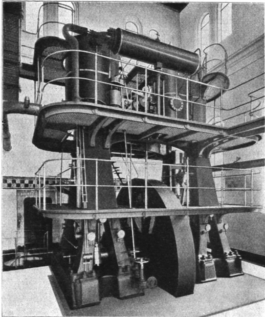
Abb. 708. Verbundmaschine VI.
