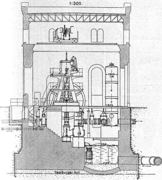
Abb. 705 und 706. Verbundmaschinen III und VIII, Schnitt und Ansicht.
