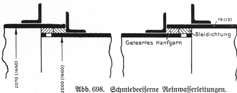
Abb. 698. Schmiedeeiserne Reinwasserleitungen.
