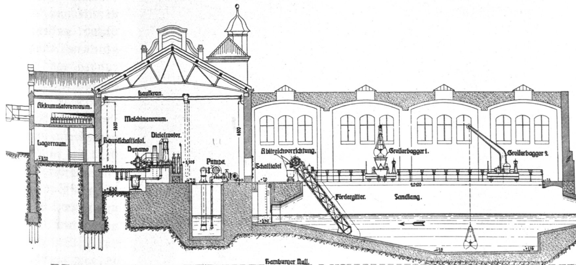
Abb. 638. Abfischanlage des südlichen Elbufers, Längenschnitt.
