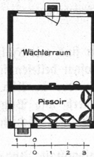
Grundriß.
