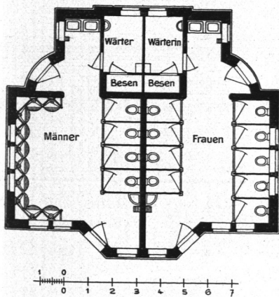
Abb. 534. Bedürfnisanstalt am Deichtor, Grundriß.
