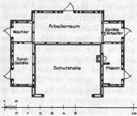
Abb. 469. Jugendspielfeld Hasselbrookstraße, Schutzhalle, Grundriß.
