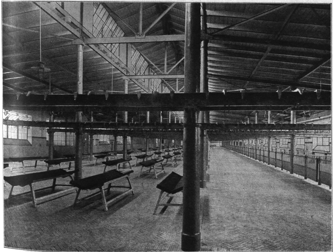
Abb. 400. Neue Schlachthalle, Kleinviehslachthalle.
