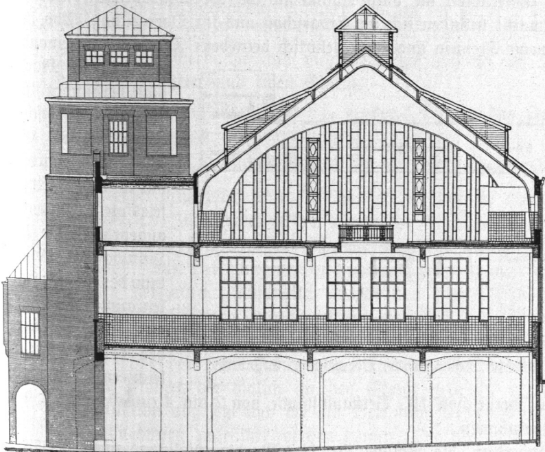
Abb. 383. Marktanlagen am Deichtor, Blumenhalle, Querschnitt.
