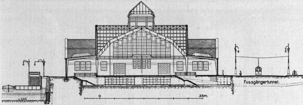
Abb. 370. Marktanlagen am Deichtor, südliche Markthalle, Schnitt.
