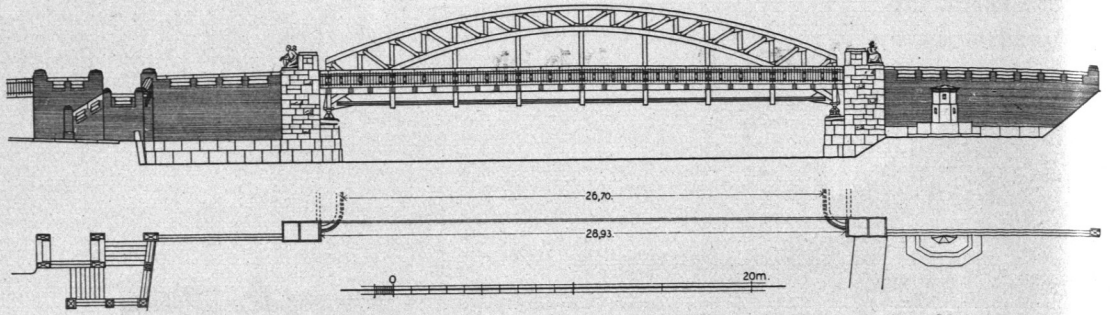
Abb. 315 und 316. Brücke Auschlägerweg, Ansicht und Brüstungsgrundriß.
