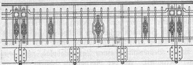
Abb. 317. Brücke Auschlägerweg, Einzelheiten des Geländers.
