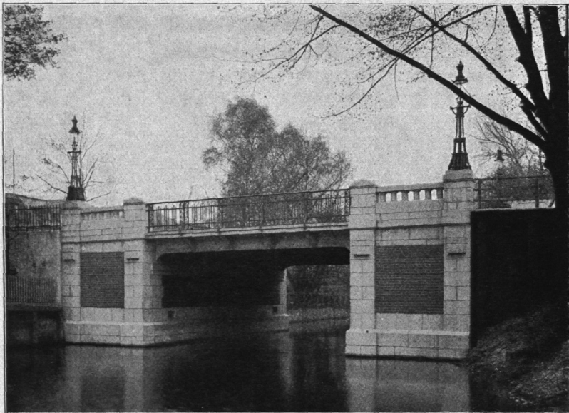
Abb. 287. Clärchenbrücke, Ansicht.
